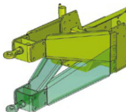
Barra de tração regulável
