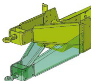
Barra de tração regulável
